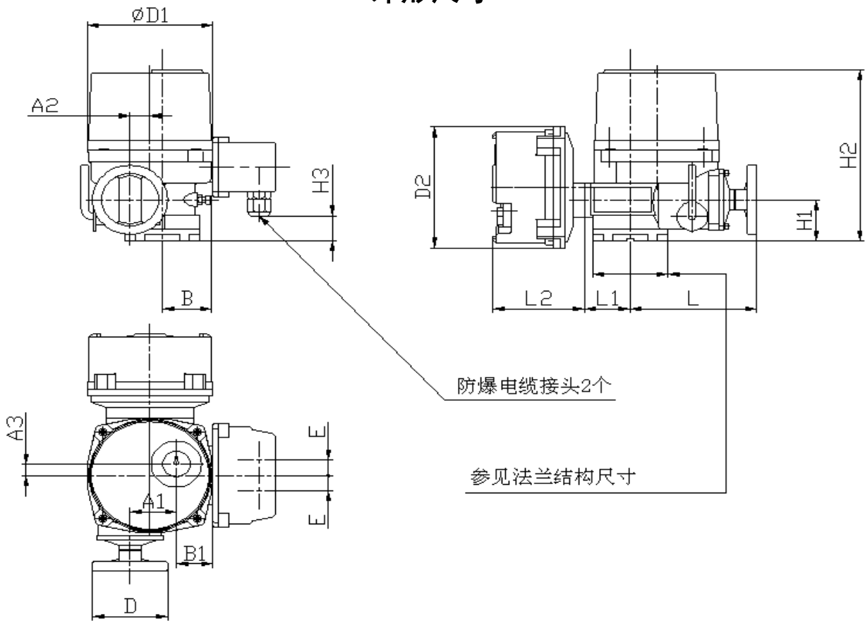
图 1 BJ 外形尺寸示意图 BJ 部分回转执行器外形尺寸
