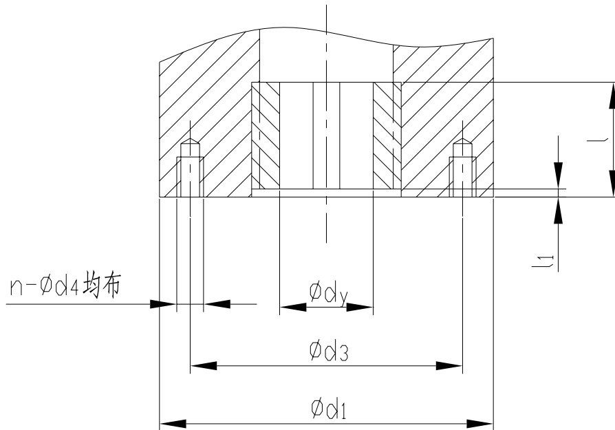
图 2 BJ 法兰连接尺寸示意图
